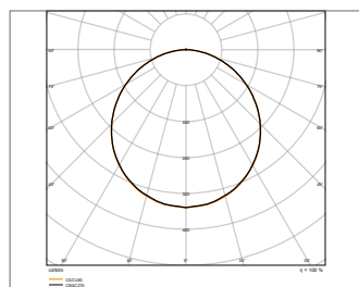
PL PROT 600 P 36W 830 PS
