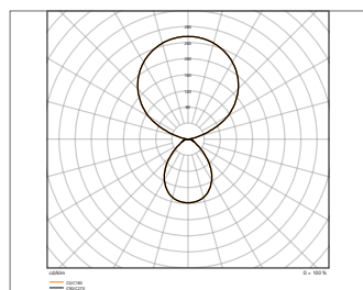
FS COMP SN EU V 88W 840 WT
